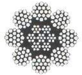
8 x 19 (W)+IWRC
